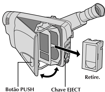
Botão PUSH
